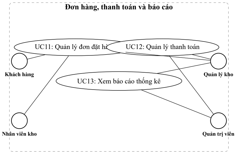
Hình 1: Sơ đồ use case phân rã – Đơn hàng, thanh toán và báo cáo
